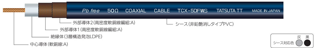
◎可動用Dタイプ同軸ケーブル「TCX-5DFWS」
