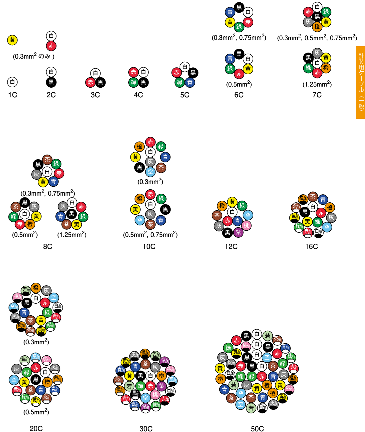
【パターン①】層撚り (C) 配列 MVVS
