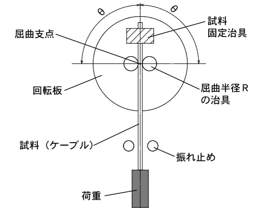
図. 一点屈曲試験
