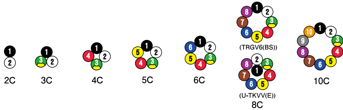
【パターン③】層燃り(C)配列 U-TKVV □C-AWG18,16
