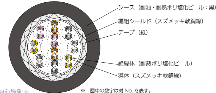
●線心識別表
