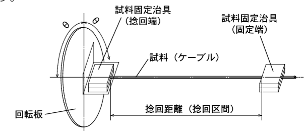
図. 捻回屈曲試験
