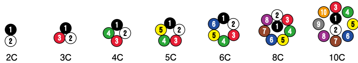
【パターン④】層燃り(C)配列 U-TKVVBS □C-AWG18,16
