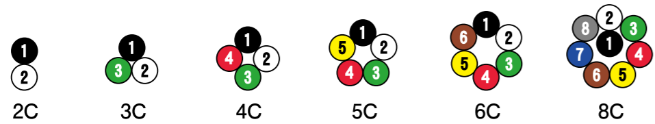
【パターン⑤】層燃り(C)配列 U-TKVV □C-AWG24,22,20、U-TKVVBS □C-AWG24,22,20
