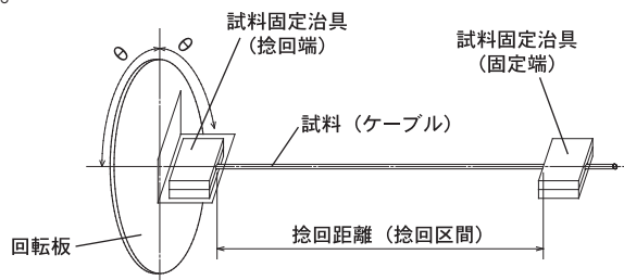
図 7-3. 捻回屈曲試験
