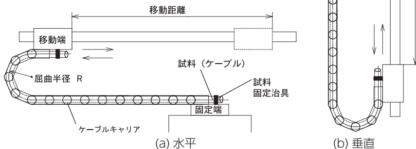
図 7-2. 移動屈曲試験
