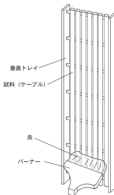
図 5-4. 垂直トレイ燃焼試験
