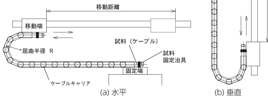
図. 移動屈曲試験
