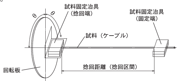
図. 捻回屈曲試験
