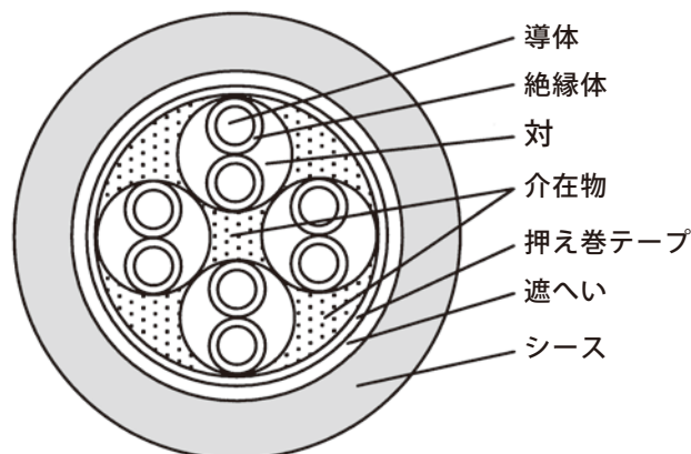
構造図
